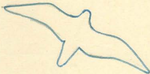
F. peregrinus.
