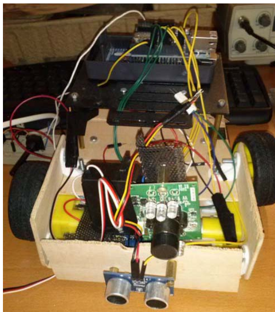
Figura 2. Sistema controlado mediante Arduino: un robot que elude obstáculos.
