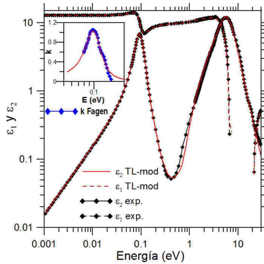
Fig. 5.6. Constante dieléctrica del SiC en función de la energía, junto con los el ajuste de TL-mod al que se le ha añadido un oscilador para incorporar también la zona de reststrahlen. En detalle, el ajuste del oscilador a los datos de k de reststrahlen de Fagen [134].
