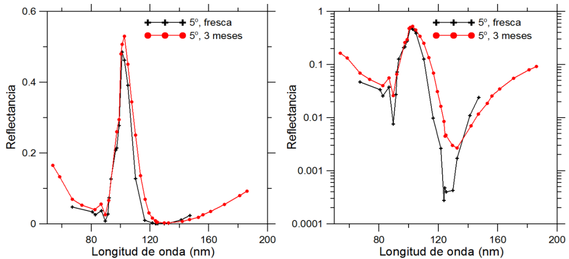
Fig. 6.6. Reflectancia a 5° en función de la longitud de onda de la muestra #3 fresca, y tras ser almacenada 3 meses en un desecador. Izquierda y derecha: reflectancia en escala lineal y logarítmica, respectivamente.
