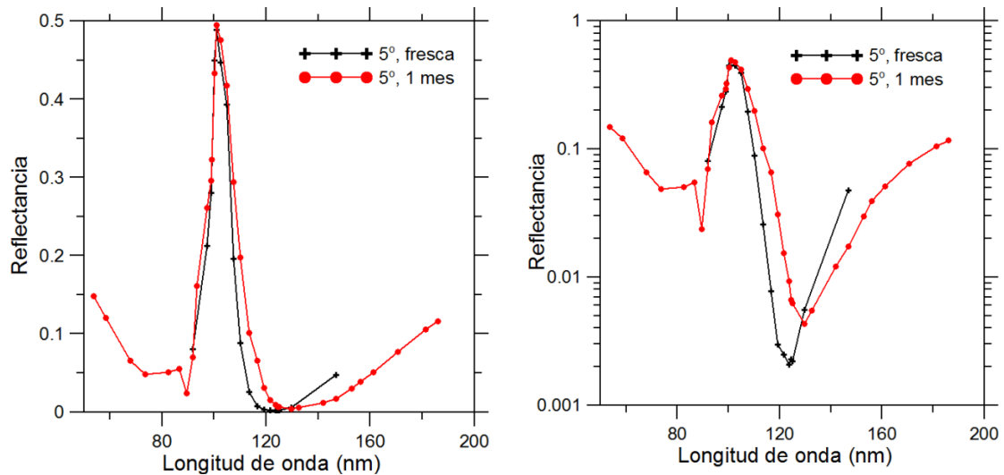
Figura. 6.5. Reflectancia a 5° en función de la longitud de onda de la muestra #2 fresca, y tras ser almacenada 1 mes en un desecador. Izquierda y derecha: reflectancia en escala lineal y logarítmica, respectivamente.
