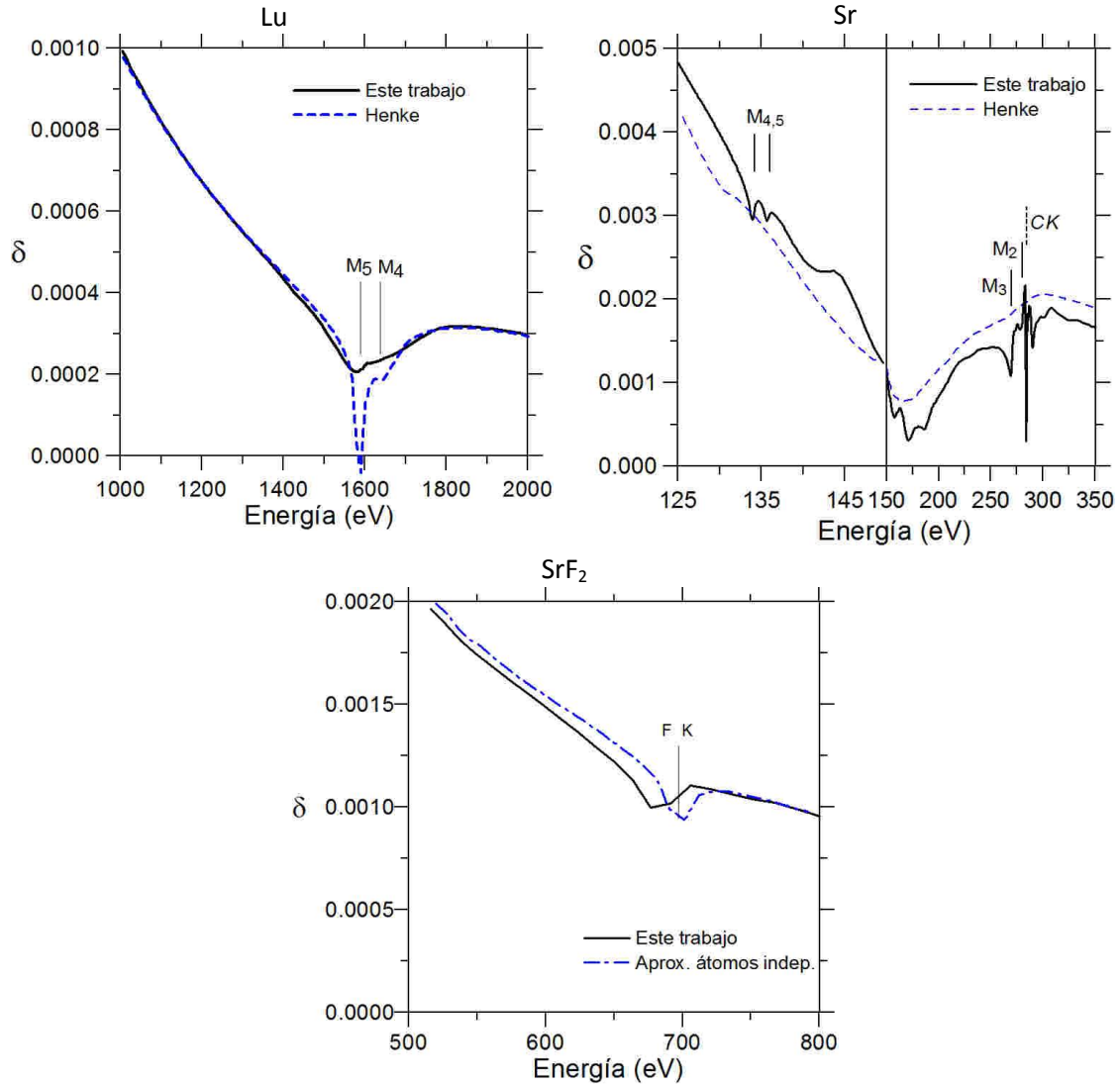
Fig. 4.9. \delta del Lu, Sr y \text{SrF}_2 para los bordes M_{4,5} del Lu, M_{4,5} y M_{2,3} del Sr y el borde K del F presente en el \text{SrF}_2 , en función de la energía de los fotones incidentes. Se compara con los datos semiempíricos de Henke et al. [101] en el caso del Lu y Sr, y con la aproximación atómica de \text{Sr}+\text{F} , para el caso del \text{SrF}_2 .
