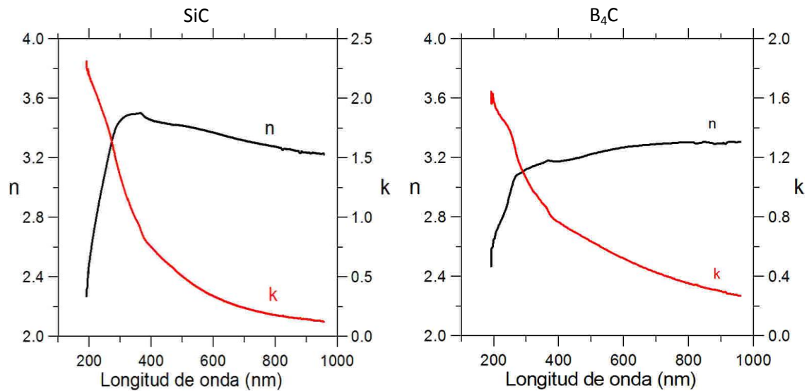
Fig. 4.11. Constantes ópticas n y k del SiC y B_4C , obtenidas a partir de las medidas de elipsometría, en función de la longitud de onda de los fotones incidentes.
