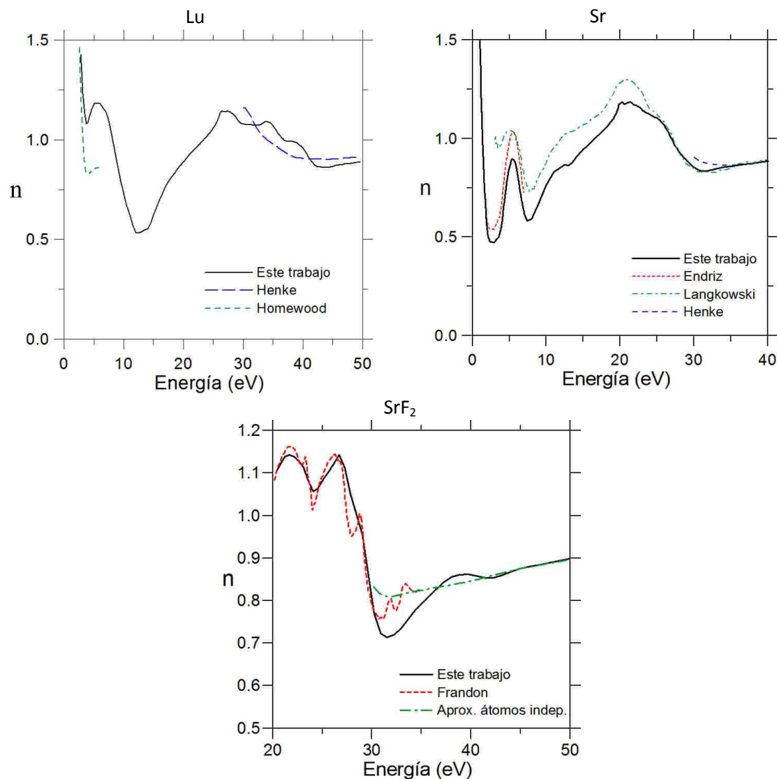
Fig. 4.8. n del Lu, Sr y \text{SrF}_2 en función de la energía de los fotones incidentes. Se compara con los datos de Homewood y Trodahl [91] y los semiempíricos de Henke et al. [101] en el caso del Lu, con Endriz y Spicer [103], Langkowski [109] y los semiempíricos de Henke et al. , en el caso del Sr y con los datos de Frandon et al. [111] y la aproximación atómica \text{Sr} + \text{F} , para el caso del \text{SrF}_2 .
