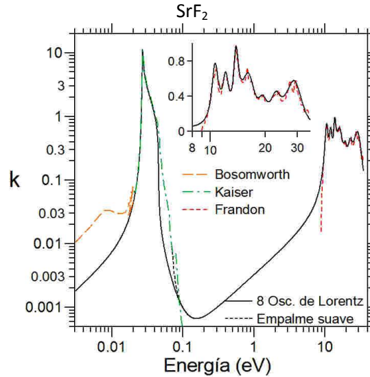
Fig. 4.5. k del \text{SrF}_2 en la zona de transparencia y zonas colindantes en función del logaritmo de la energía de los fotones incidentes, junto con el ajuste de ocho osciladores de Lorentz a los datos experimentales de Frandon et al. [111] y Kaiser et al. [122], y los datos de Bosomworth [123].
