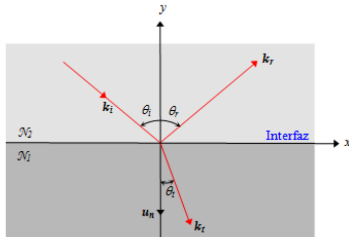
Figura. 2.1. Onda plana incidente en la frontera entre dos medios homogéneos e isótropos.
