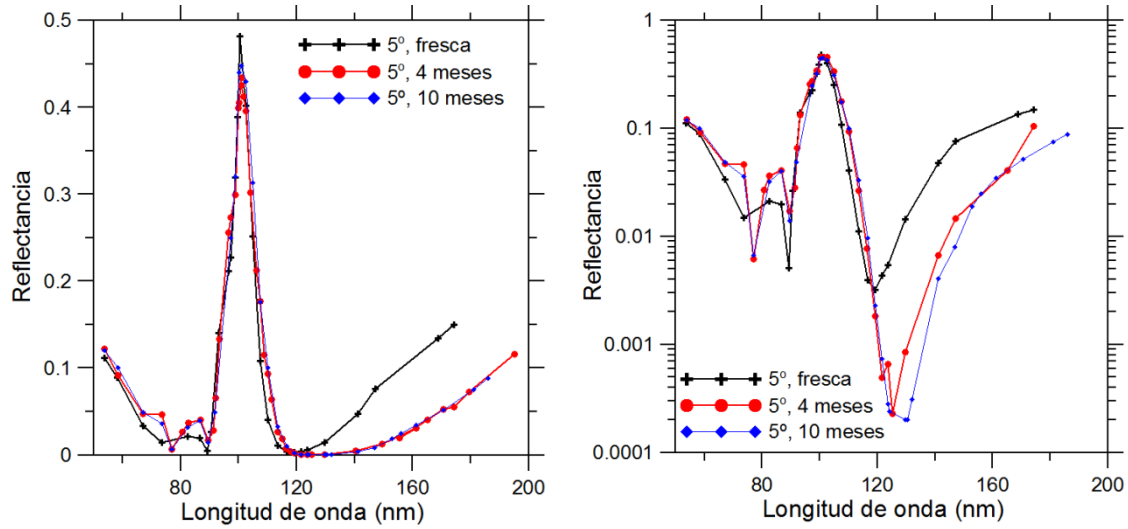
Fig. 6.4. Reflectancia a 5° en función de la longitud de onda de la muestra #1 fresca, y tras ser almacenada 4 meses y 10 meses en un desecador. Izquierda y derecha: reflectancia en escala lineal y logarítmica, respectivamente.
