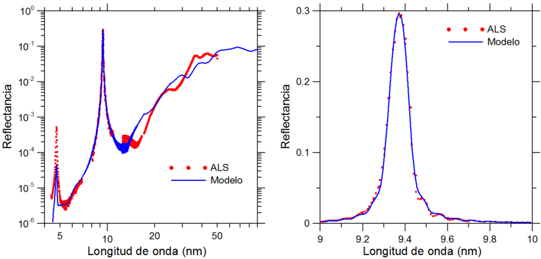
Fig. 6.24. Reflectancia a 3° experimental (rojo) y el modelo (azul) en función de la longitud de onda para la multicapa de Mo/Y centrada en 9.39 nm. A la izquierda, ajuste en banda y fuera de banda. A la derecha, ajuste en banda.
