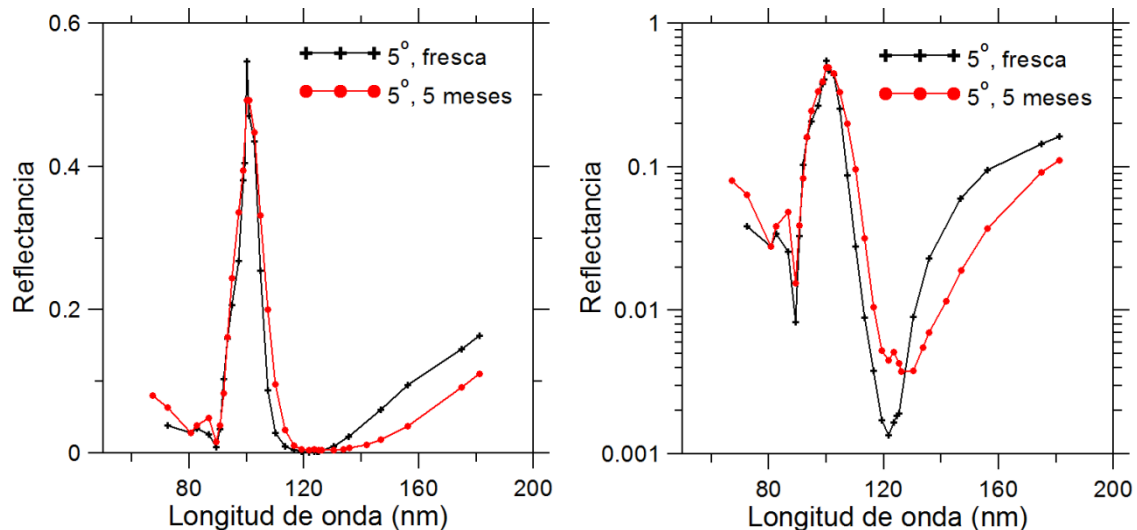
Fig. 6.7. Reflectancia a 5° en función de la longitud de onda de la muestra #4 fresca, y tras ser almacenada 5 meses en un desecador. Izquierda y derecha: reflectancia en escala lineal y logarítmica, respectivamente.
