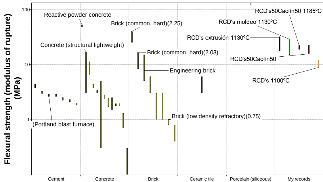
Figura 133: Comparación de la resistencia a flexión de los materiales estudiados con los materiales cerámicos tradicionales [305].
