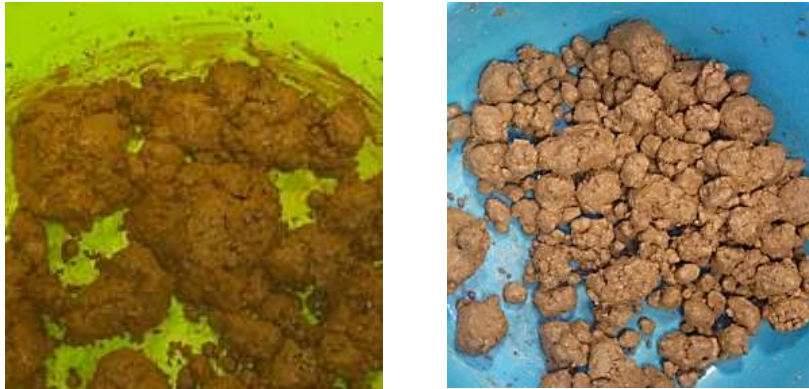
Figura 42: Amasado de las mezclas a) RCD's y b) 50% RCD's + 50% caolín.
