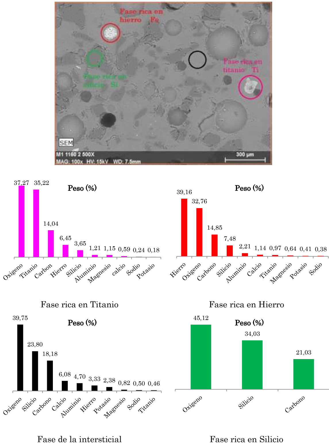
Figura 110: Microestructura e identificación de las fases en las piezas sinterizadas a 1160°C.
