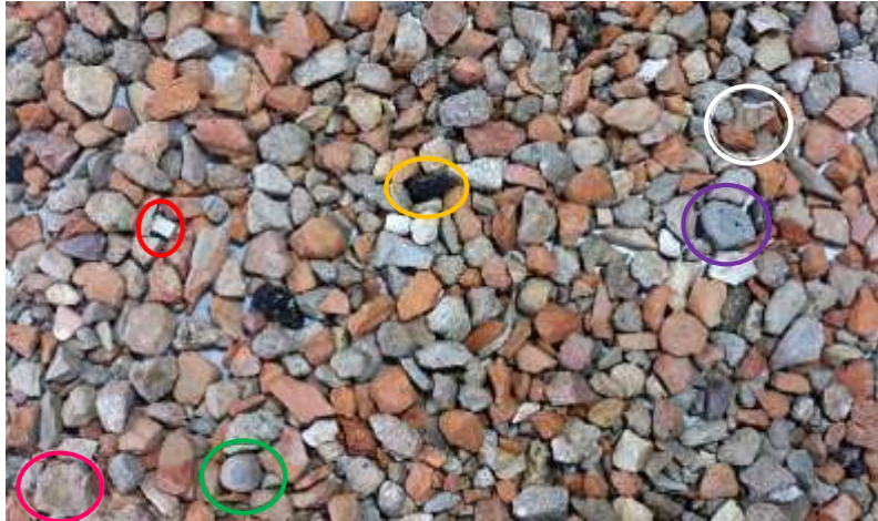
Figura 20: Tanda de RCD's indicando: ladrillo, mortero, hormigón, loza y alquitrán.
