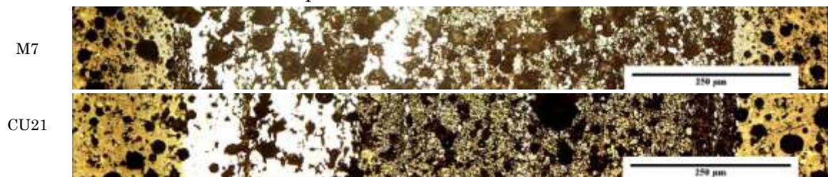
Figura 157: Barridos microscópicos del ancho de pista a 1000x, moldeo, compactación y extrusión.
