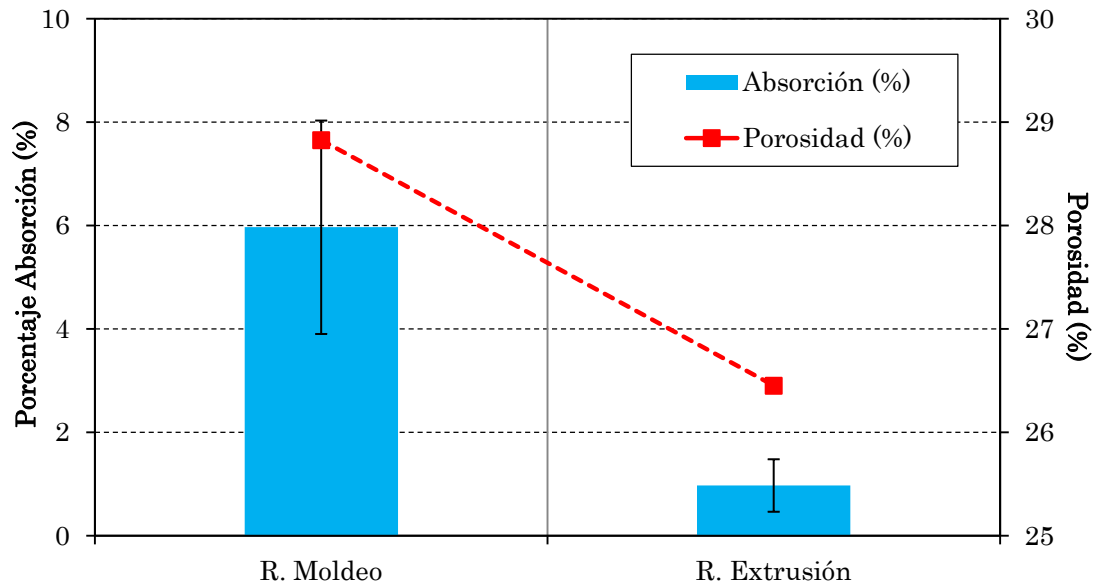
Figura 137: Porcentaje de absorción media de las piezas moldeadas y extruidas sinterizadas a 1130°C.
