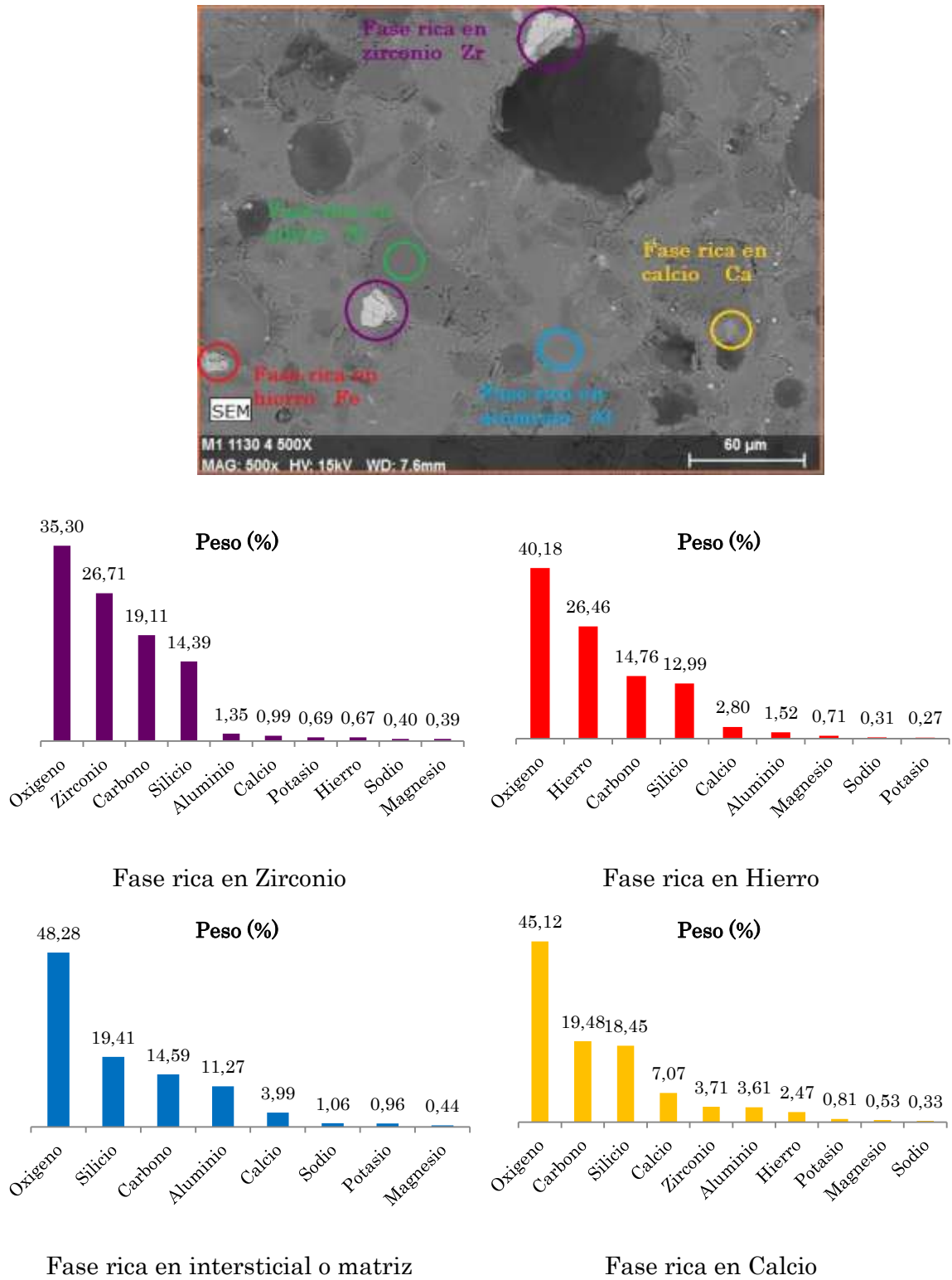
Figura 109: Microestructura e identificación de las fases en las piezas sinterizadas a 1130°C.
