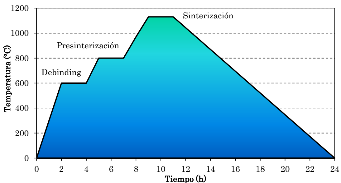
Figura 47: Ejemplo del ciclo térmico de sinterización seguido.
