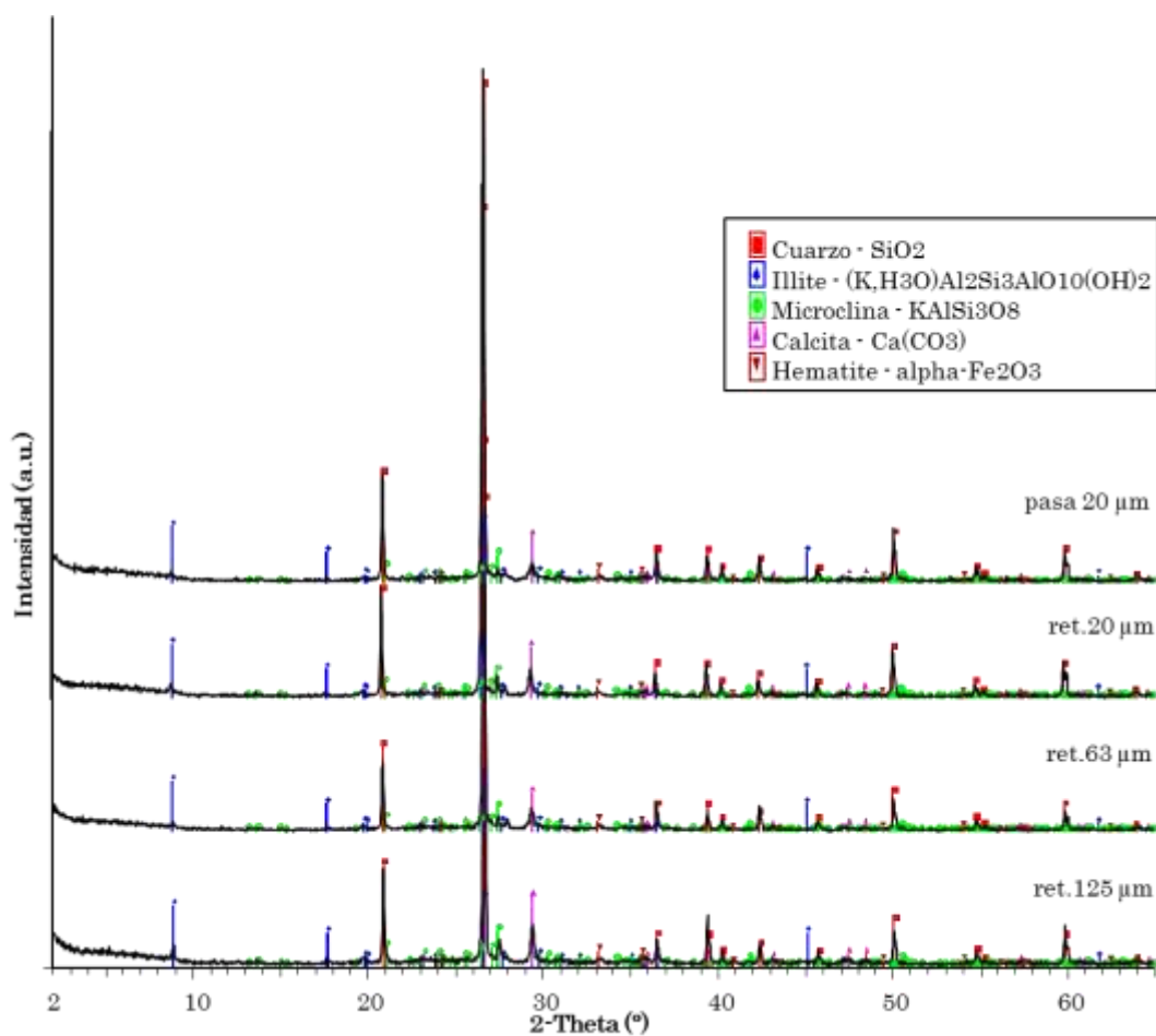
Figura 85: DRX de los RCD's retenido en los tamices #125 µm, # 63 µm, # 20µm y pasa #20 µm.
