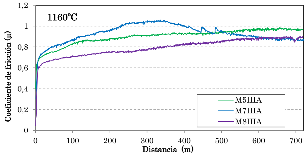
Figura 207: Coeficientes de fricción para las piezas moldeadas y sinterizadas a 1160°C.
