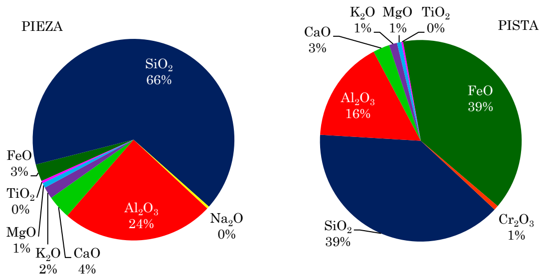
Figura 198: a) Composición química de la pieza y b) composición química de la pista de desgaste.
