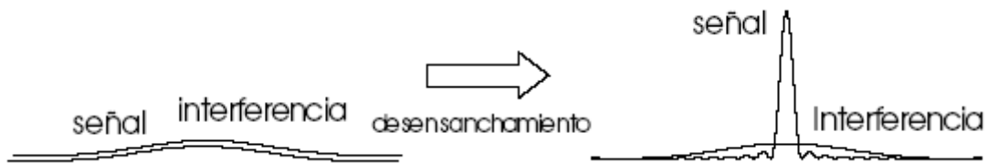
Figura 0.83: Protección contra interferencias de banda ancha
