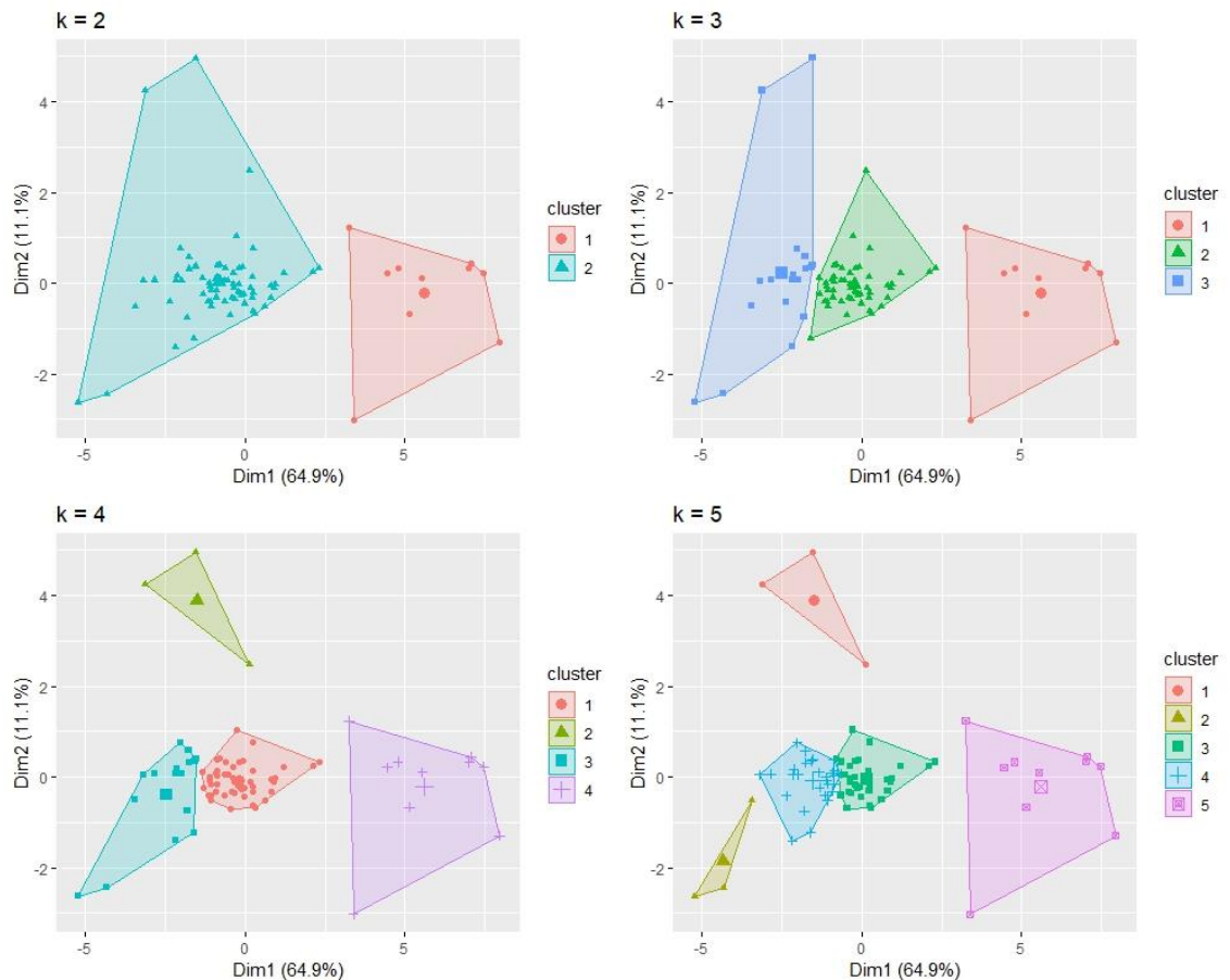
Figura 17: Diagramas de análisis de 2, 3, 4 y 5 clusters ( k=1 , k=2 , k=3 , k=4 , k=5 ) con representación de los resultados en dos dimensiones (Dim) que engloban el 76 % de la variabilidad de los datos de la muestra estandarizados (Dim 1: 64.9%, Dim 2: 11.1%). Análisis de clasificación en 2 clusters ( k=2 , arriba izquierda), 3 clusters ( k=3 , arriba derecha), 4 clusters ( k=4 , abajo izquierda) o 5 clusters ( k=5 , abajo derecha).
