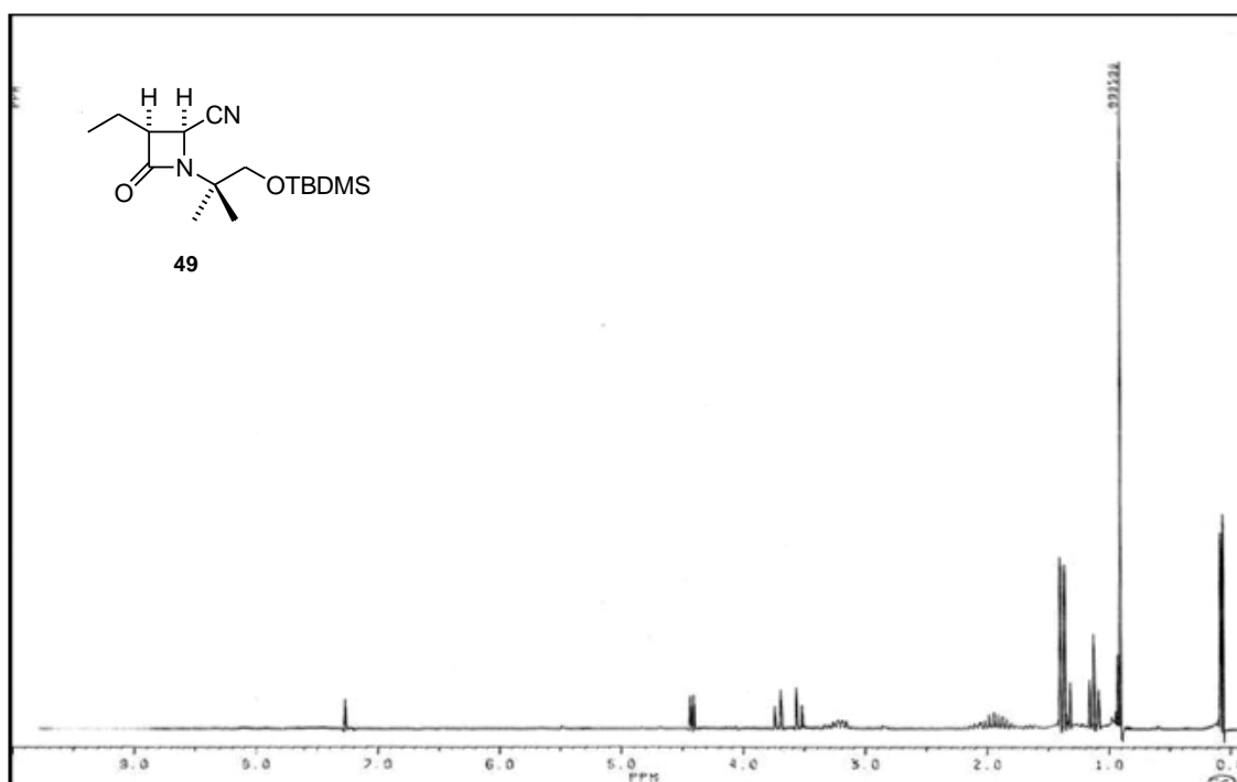
Espectros RMN ^1\text{H} , RMN ^{13}\text{C} e IR del compuesto 49
