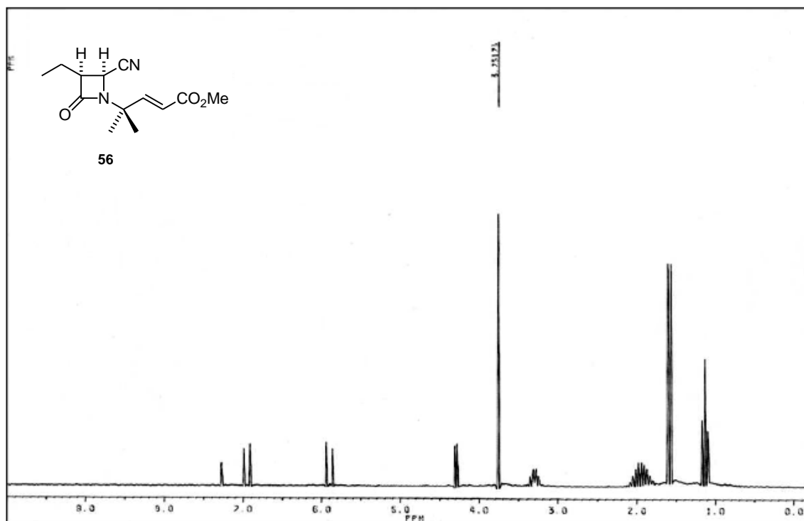
Espectros RMN ^1\text{H} , RMN ^{13}\text{C} e IR del compuesto 56
