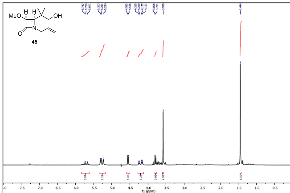
Espectros RMN 1 H, RMN 13 C e IR del compuesto 45
