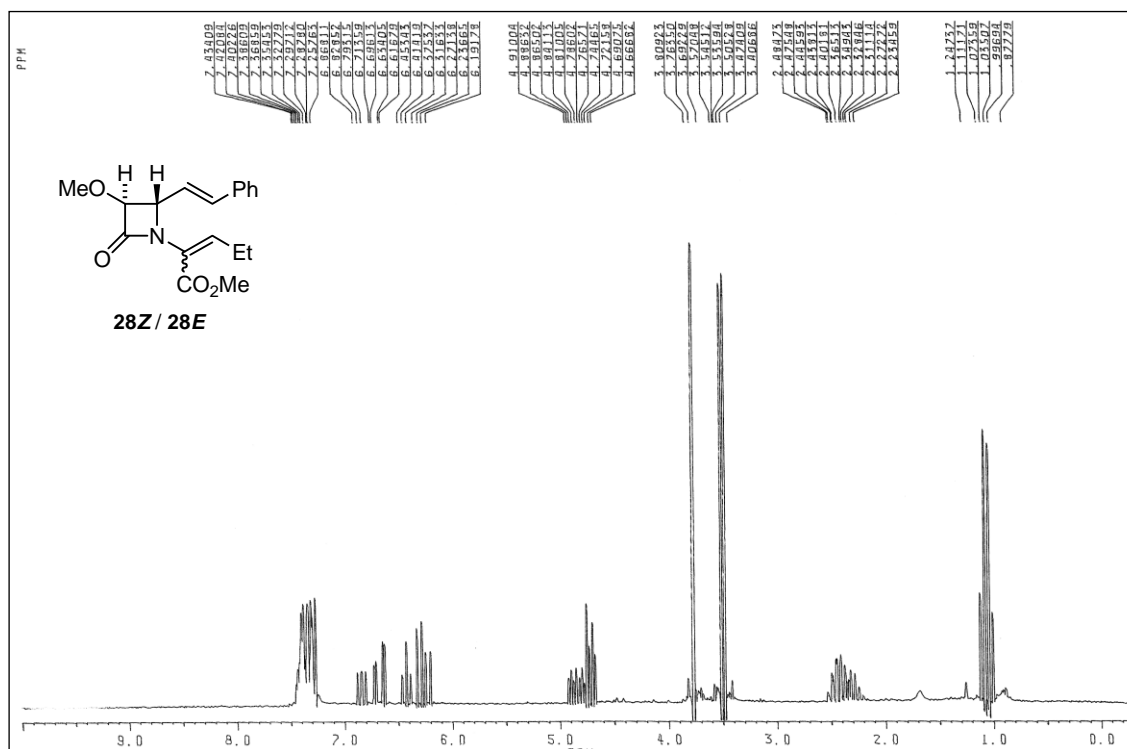
Espectros RMN 1 H, RMN 13 C, e IR de una mezcla de los diastereoisómeros 28Z y 28E
