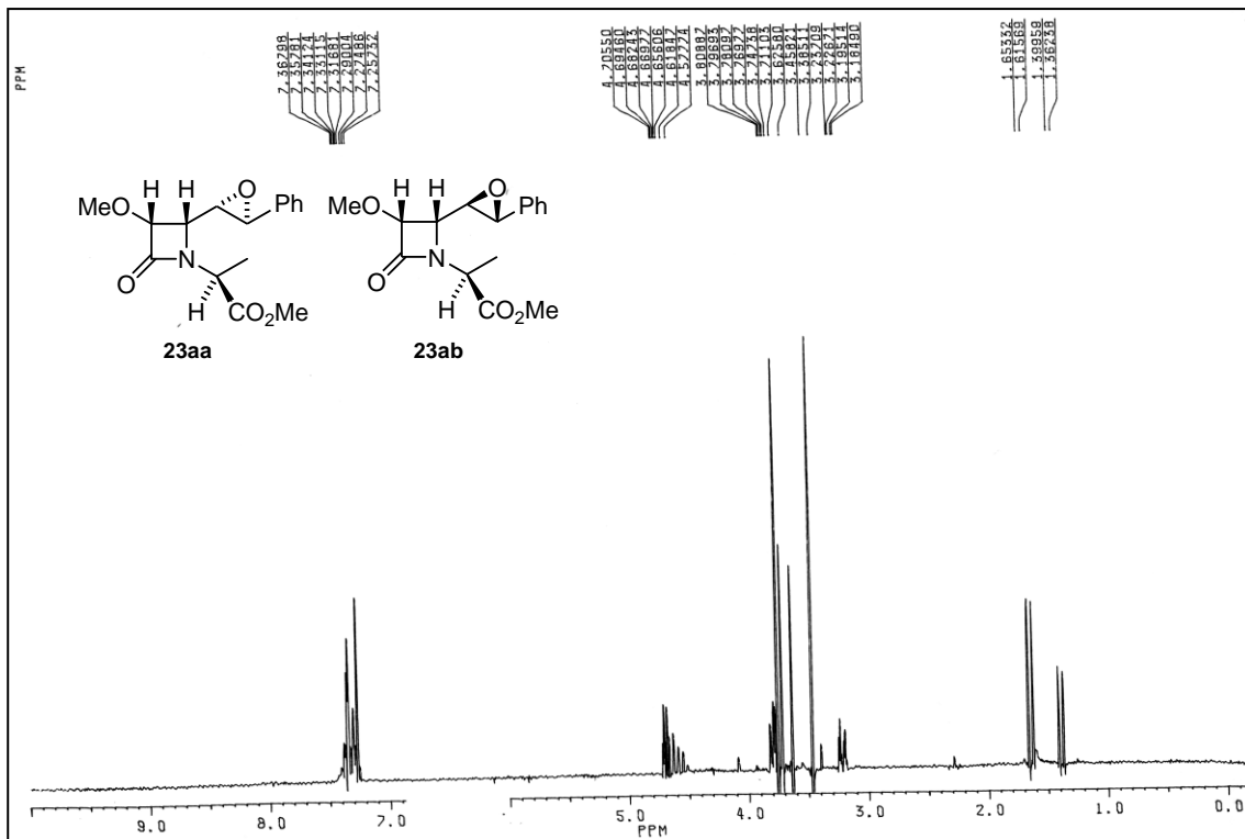
Espectro RMN 1 H de una mezcla de los compuestos 23aa y 23ab
