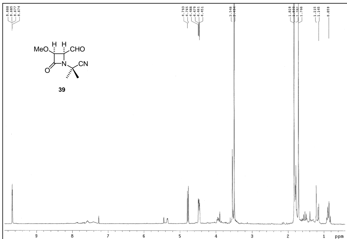
Espectros RMN- 1 H y RMN 13 C del compuesto 39
