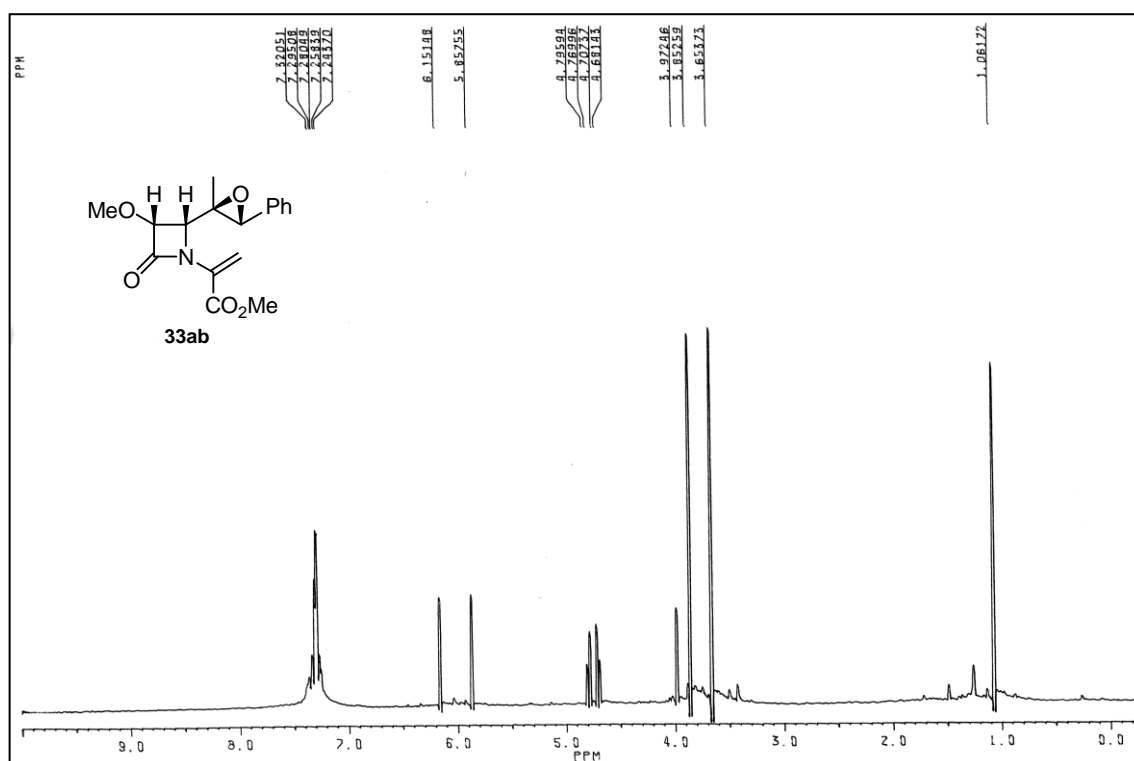
Espectros RMN ^1\text{H} , RMN ^{13}\text{C} e IR del compuesto 33ab
