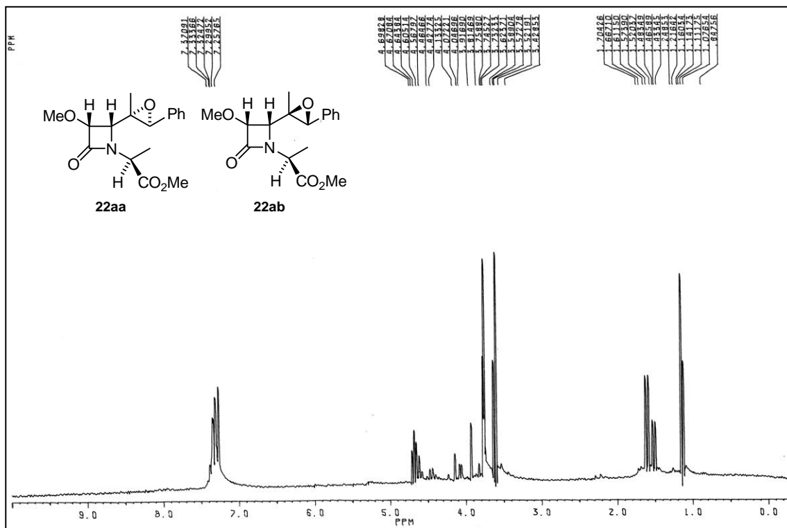
Espectro RMN 1 H de una mezcla de los compuestos 22aa y 22ab
