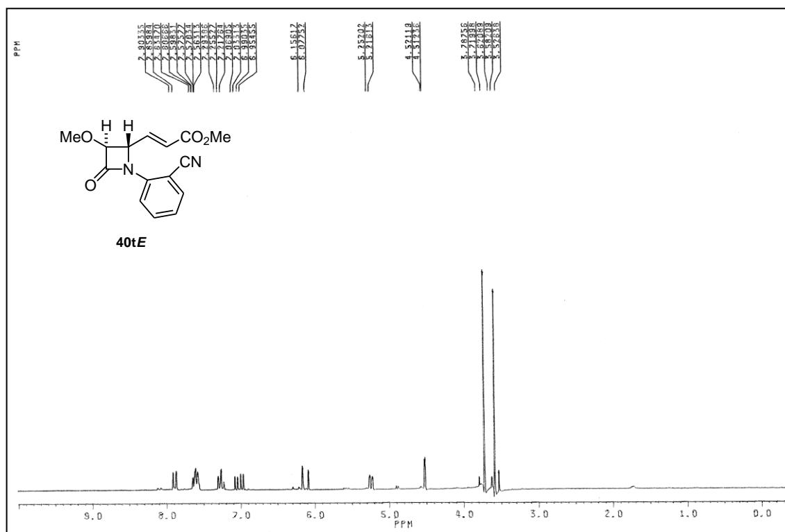
Espectro RMN 1 H del compuesto 40tE
