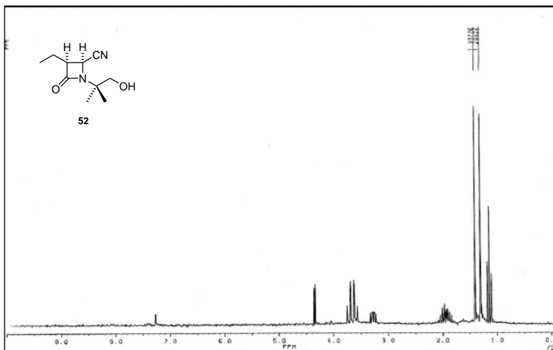
Espectros RMN 1 H, RMN 13 C e IR del compuesto 52
