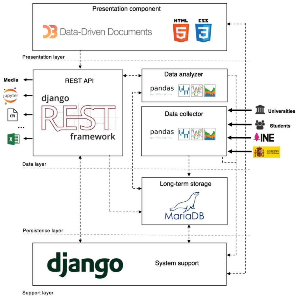
Figura 7. Tecnologías utilizadas en el ecosistema del OEEU
