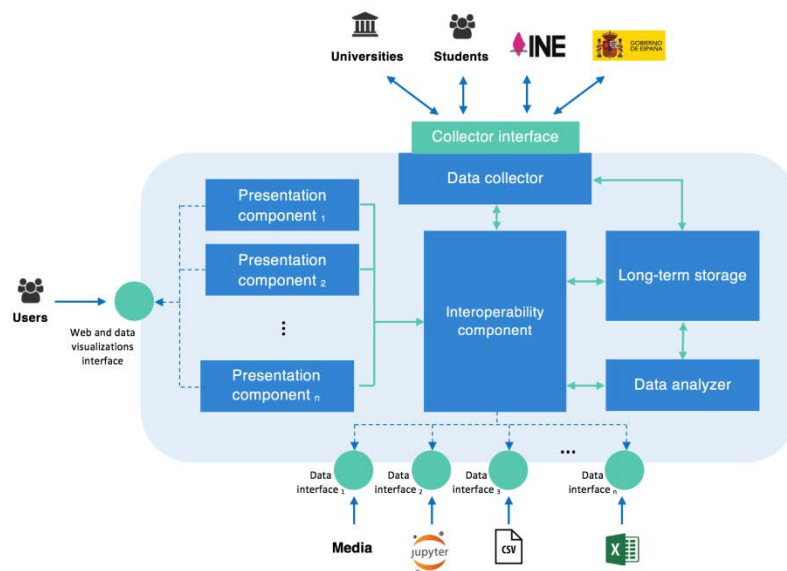
Figura 6. Esquema del ecosistema tecnológico del Observatorio de Empleabilidad y Empleo Universitario
