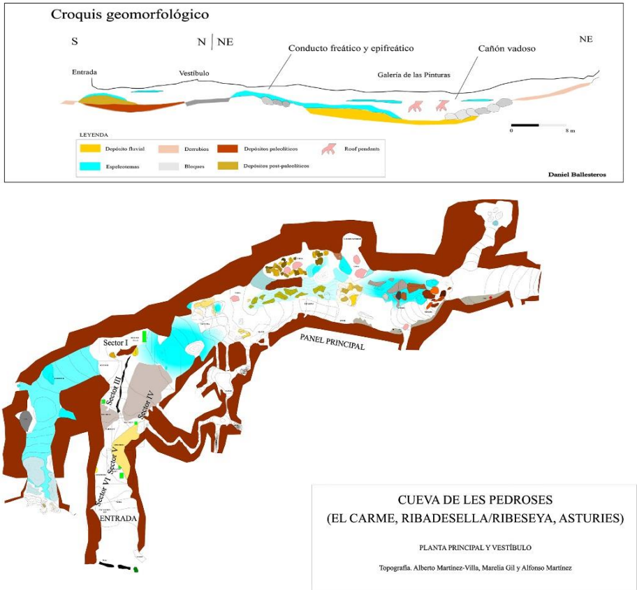
Figura 5. Planta topográfica. Galería principal y croquis geomorfológico.
