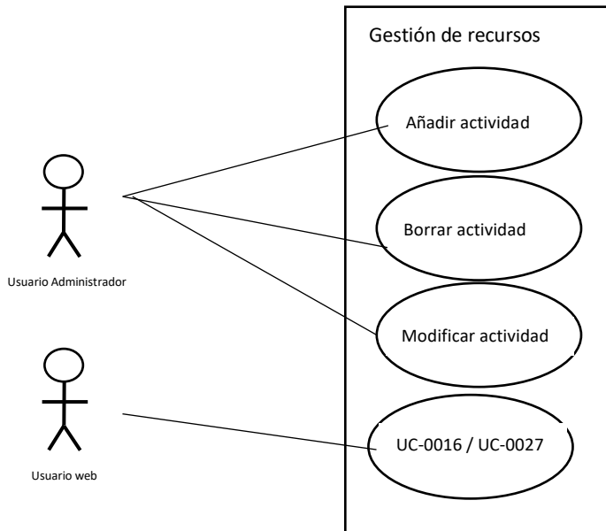
Figura 6. Diagrama de casos de uso. Gestión de recursos
