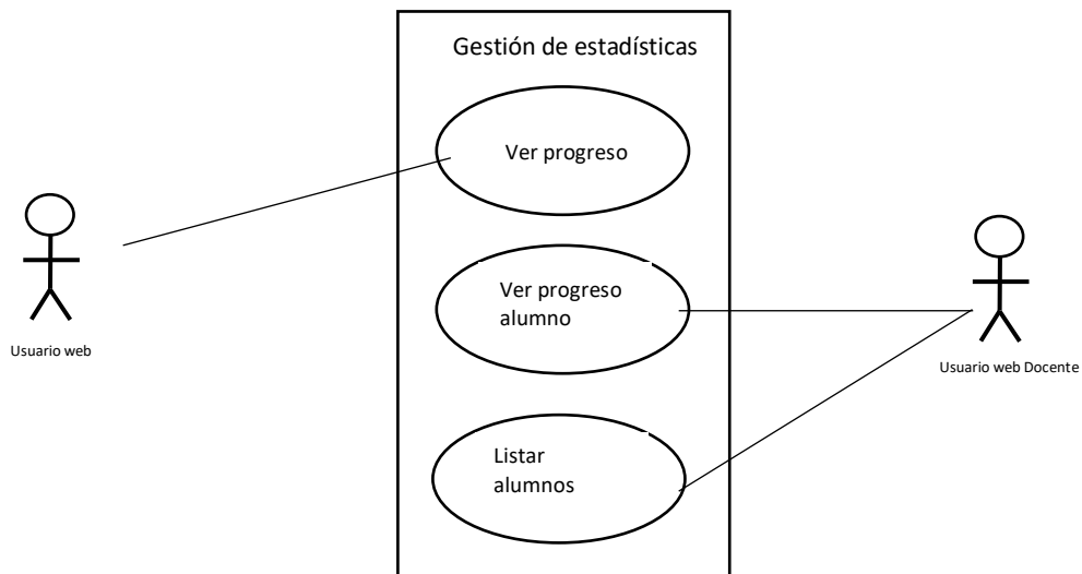
Figura 4. Diagrama de casos de uso. Gestión de estadísticas
