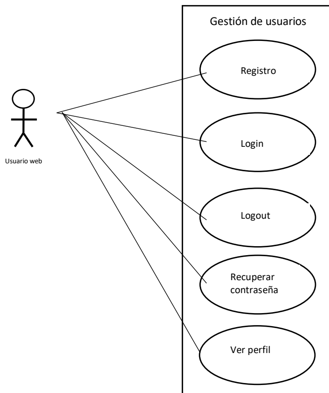
Figura 3. Diagrama de casos de uso. Gestión de usuarios
