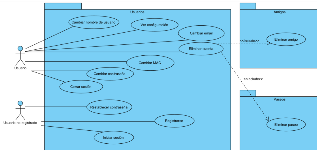
Figura 2. Diagrama de casos de uso- Usuarios.
