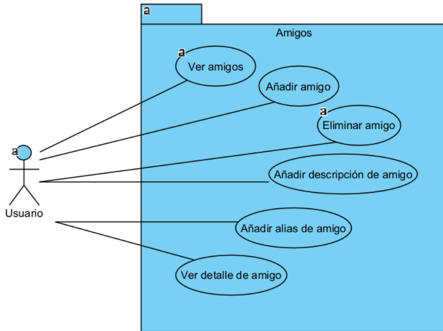
Figura 4. Diagrama de casos de uso- Amigos.
