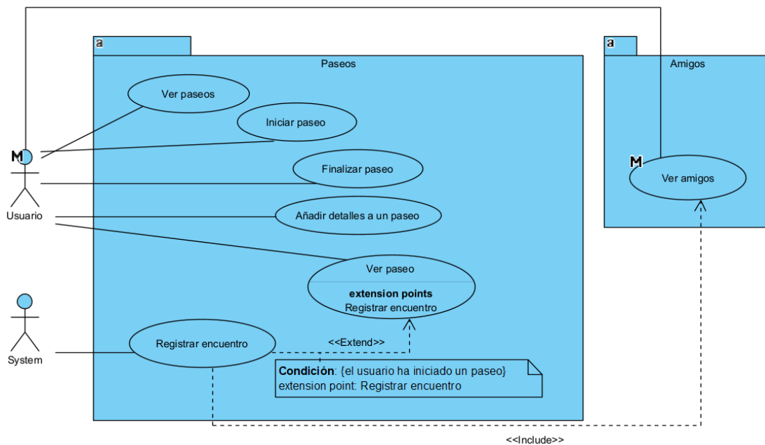
Figura 3. Diagrama de casos de uso- Paseos.
