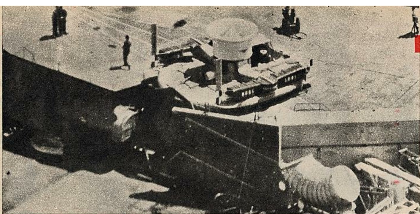
Una foto «histórica» en materia de aeronaves de planta circular. El prototipo del «Hovercraft» construido por la Saunders Roe, fotografiado el día de su primer vuelo. A este modelo han seguido otros de forma y dimensiones distintas, que sin embargo no han encontrado aceptación porque los vehículos de cojín de aire pueden aterrizar solo sobre superficies lisas
