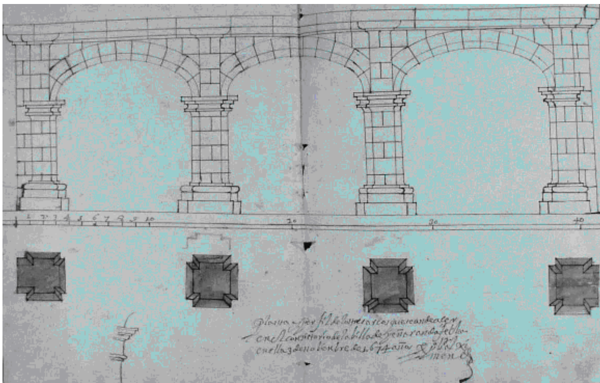
Figura 1: Planta y perfil de los tres arcos de la obra del Ayuntamiento, año 1674. (A. Histórico Provincial de Salamanca, Protocolos , 2756, f. 81 ter.)
