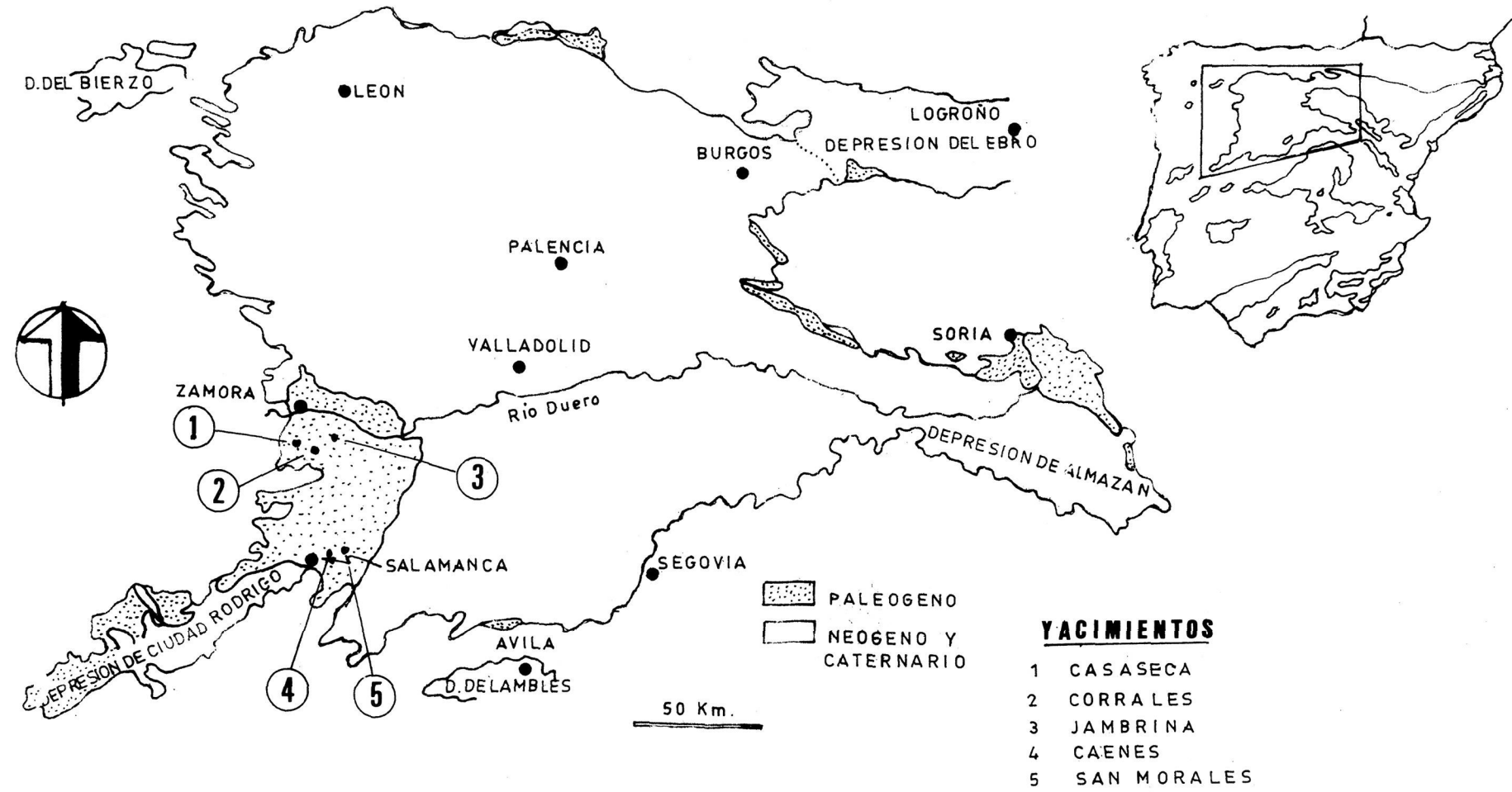
Figura 1: Localización geográfica de los yacimientos de la Cuenca del Duero (Castilla y León, España) con Lophiodontidae.
