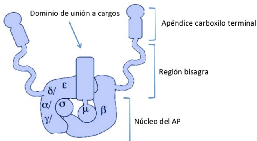
Figura 9. Estructura de los complejos AP. Estructura general de los complejos de la familia de adaptadores de clatrina AP. Se muestran las posiciones relativas de las cuatro subunidades que los componen y algunos de los dominios implicados en su función. Figura modificada de Hirst et al , 2011.
