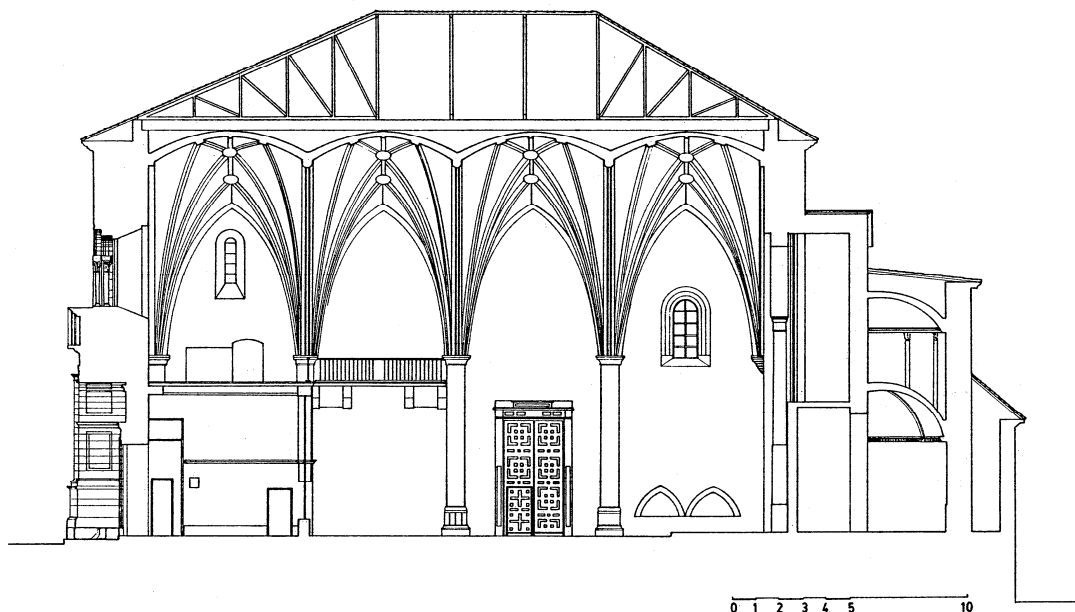
Figura 7: Iglesia de San Ildefonso, en Zamora. Sección longitudinal. Fuente: Enciclopedia del románico en Castilla y León. Zamora , p. 430. Autor: Juan Ildefonso González García
