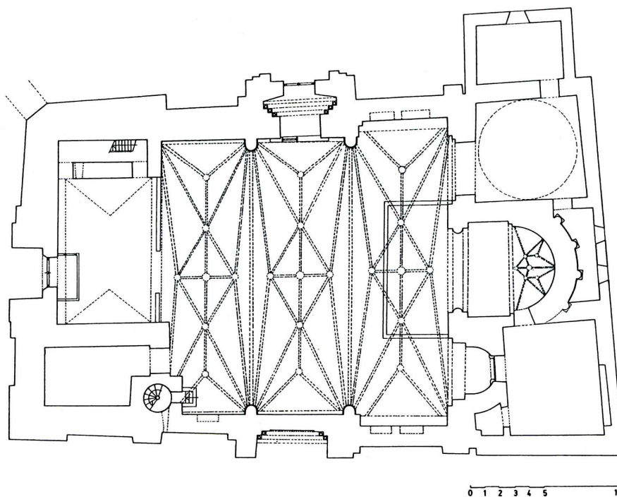
Figura 5: Iglesia de San Ildefonso, en Zamora. Planta. Fuente: Enciclopedia del románico en Castilla y León. Zamora , p. 428. Autor: Juan Ildefonso González García
