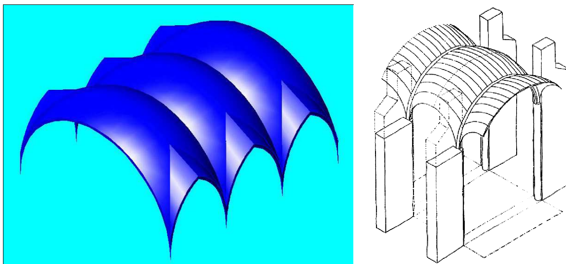
Figura 8: Iglesia de San Ildefonso, en Zamora. Modelización de las bóvedas. Fuente: Autor.
