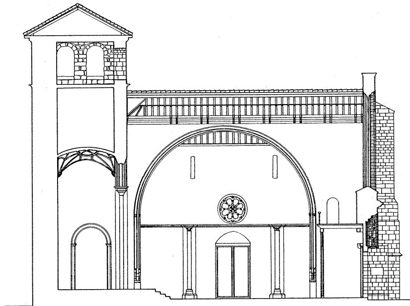
Figura 19: Iglesia de San Juan, en Zamora. Sección longitudinal. Fuente: Enciclopedia del románico en Castilla y León. Zamora , p. 462. Autor: Juan Ildefonso González García
