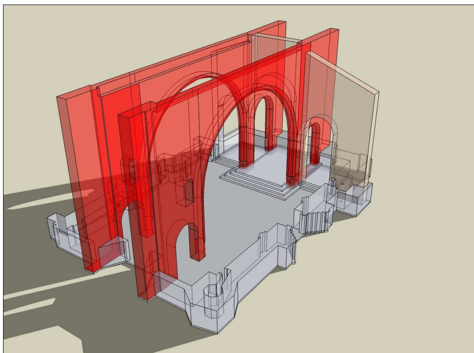
Figura 25: Iglesia de San Juan, en Zamora. Modelización de los arcos formeros. Fuente: Autor.
