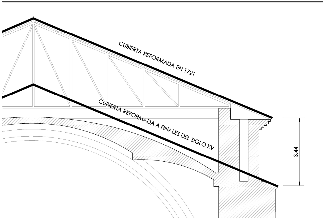
Figura 14: Iglesia de San Ildefonso, en Zamora. Sección transversal. Fuente: Autor.
