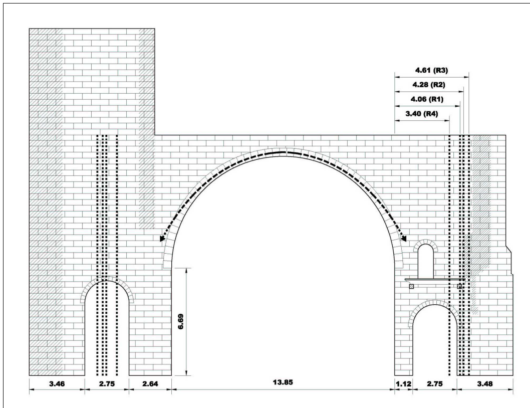
Figura 26: Iglesia de San Juan, en Zamora. Arco formero del lado de la epístola con espesores de estribo resultantes de las reglas de Gil de Hontañón. Línea de empujes. Fuente: Autor.
