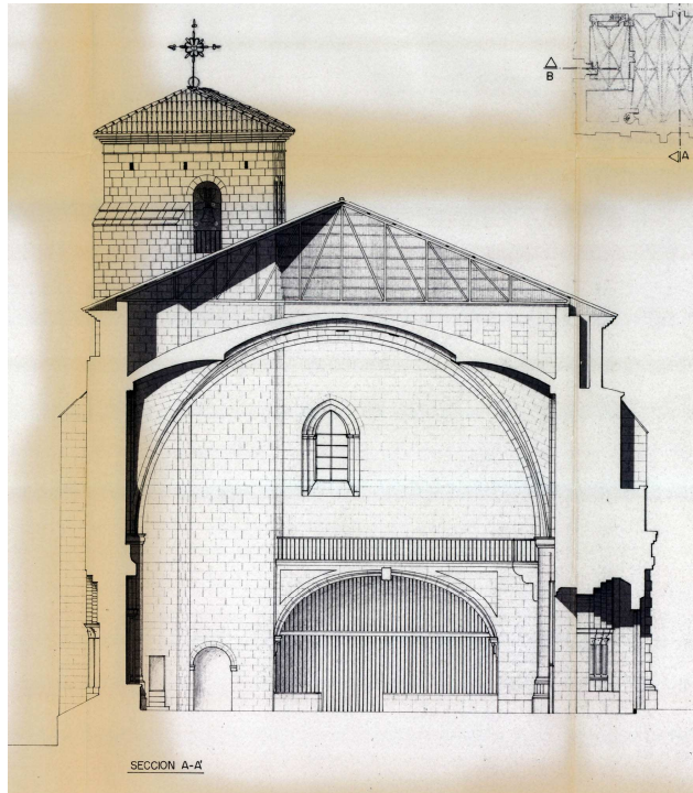
Figura 6: Iglesia de San Ildefonso, en Zamora. Sección transversal. Fuente: M.A. Lera y L.J. Peláez, Restauración 2ª fase de la iglesia de San Ildefonso (1990).
