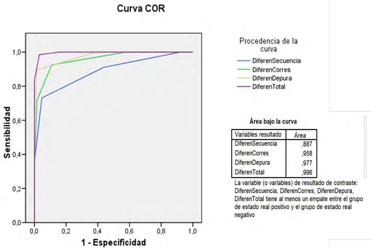
Figura 5.7 Curva ROC sobre las diferencias pretest-postest (grupo experimental)
