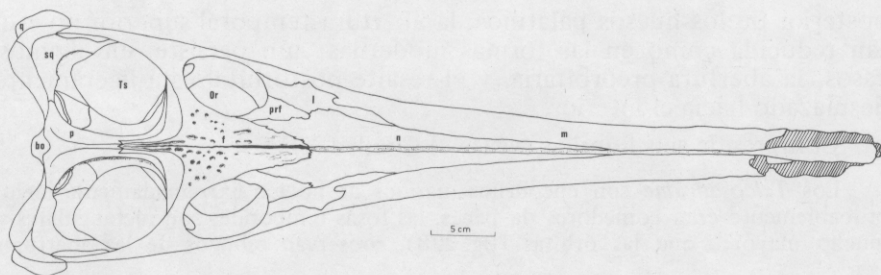
Fig. 230. Cráneo de Mystriosaurus cf. bollensis (Jaeger), un mesosúquido (Teleosauridae) del Lías de Tomar (Portugal). (Según Telles Antunes, dibujado por E. Jiménez) ( \times 0,17 .)
