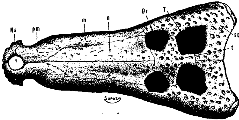
Fig. 232. Cráneo de Goniopholis crassidens , un cocodrilo de 2 m de largo del Weald de Inglaterra. T, fosa temporal súpera; las demás abreviaturas como en la fig. 162. (x 0,3; según Owen.)
