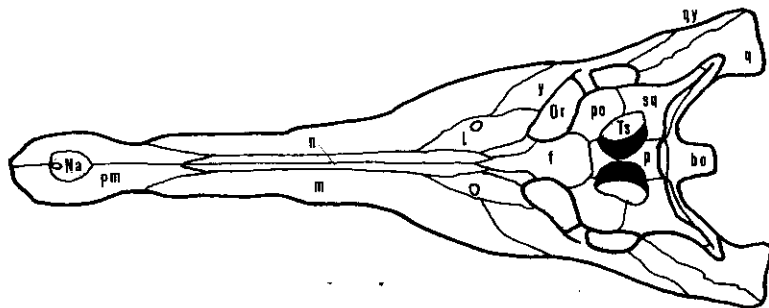
Fig. 237. Cráneo de Tomistoma lusitanica (Vianna y Moraes), del Mioceno de Portugal. (x 0,1; según Tellès Antunes, dibujado por E. Jiménez.)
