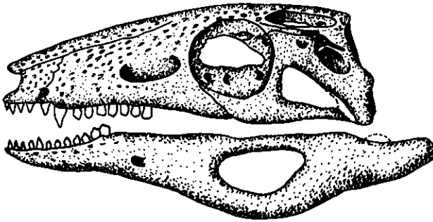
Fig. 233. Cráneo y mandíbula de Uruguaysuchus aznarensis Rusconi, del Cretácico de Uruguay. (x 0,5; según C. Rusconi, copiado por E. Jiménez.)
