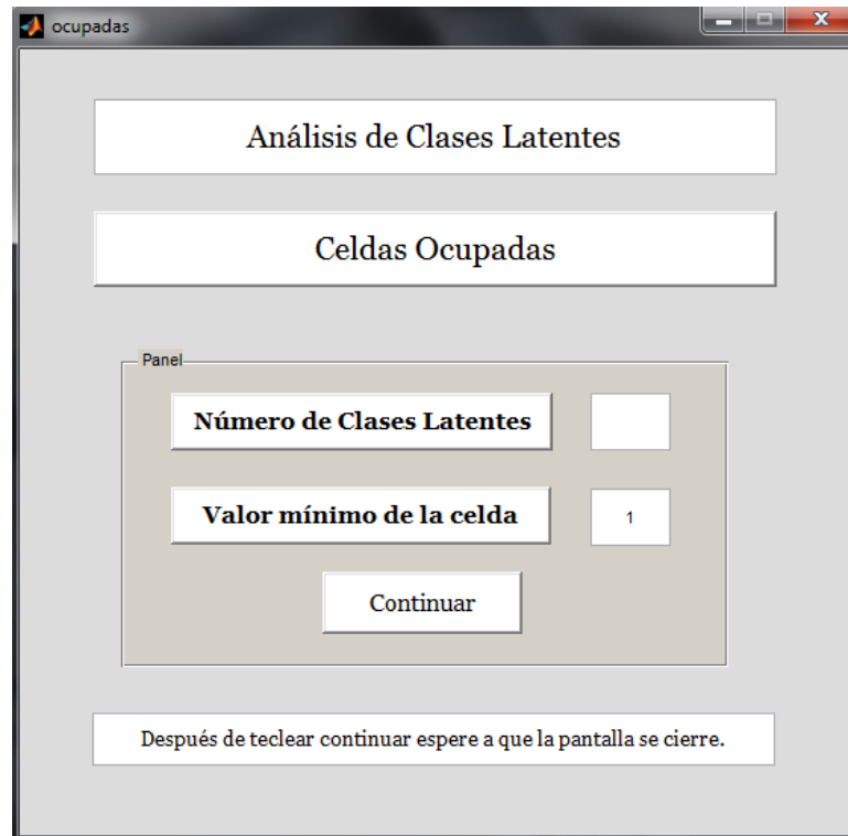
Figura 5.5. Entrada de datos a la rutina de clases latentes utilizando celdas con ocupadas.
